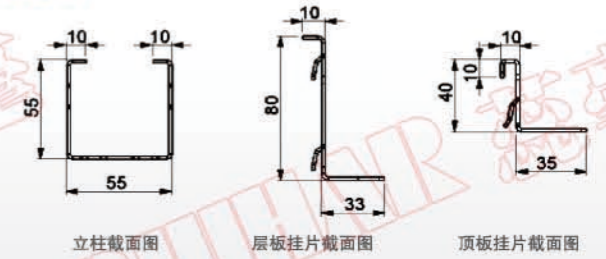
立柱截面图
